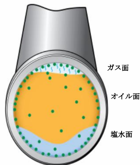
パイプラインの断面で、活性のあるVpCI防錆保護が、液面、接触面、空洞面の3界面に渡る事が示されています。
